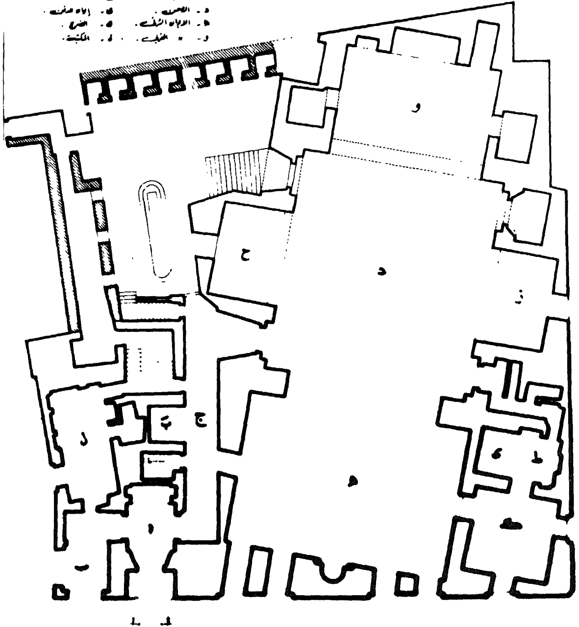
شكل ( ٦ ) يبين مسقط أفقى لدرسة الاشراف برسباى بشارع المعز لدين الله بالقاهرة
